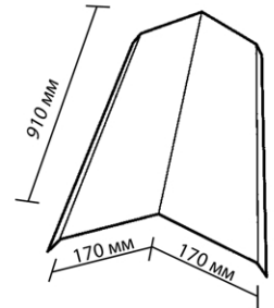
Ребровый конек
