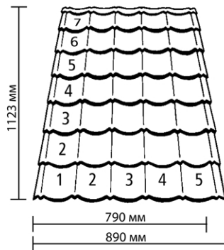
Лист Аквапан (7x5 плиток)
